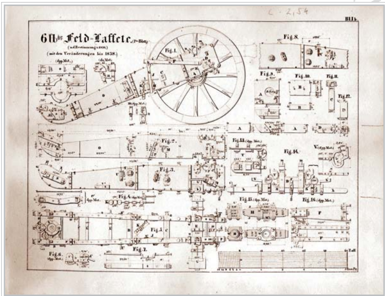
Hatfontos löveg ágyútalpának rajza
